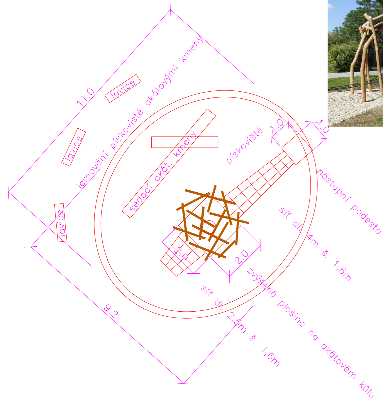
HERNÍ PRVEK "VRABČÍ HNÍZDO"
