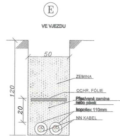
ŘEZY ULOŽENÍ KABELŮ NN-0,4kV
